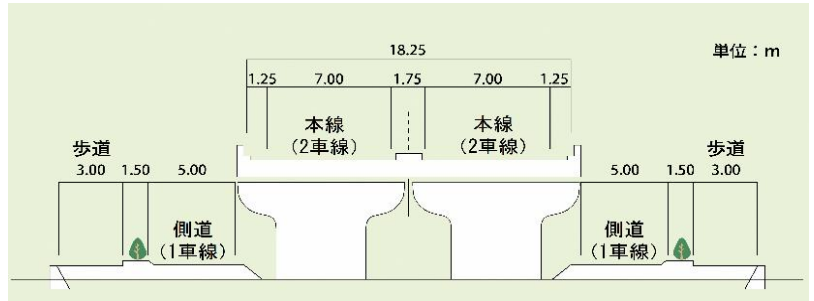
【代表断面図】国土交通省近畿地方整備局 滋賀国道事務所より
