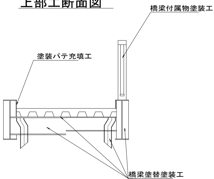
上部工断面図
