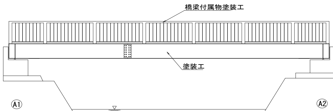
側面図
