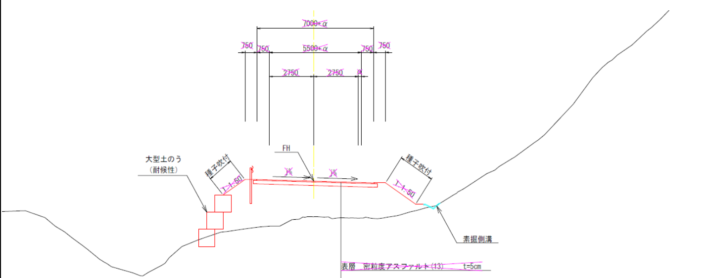
標準断面図(盛土部)
