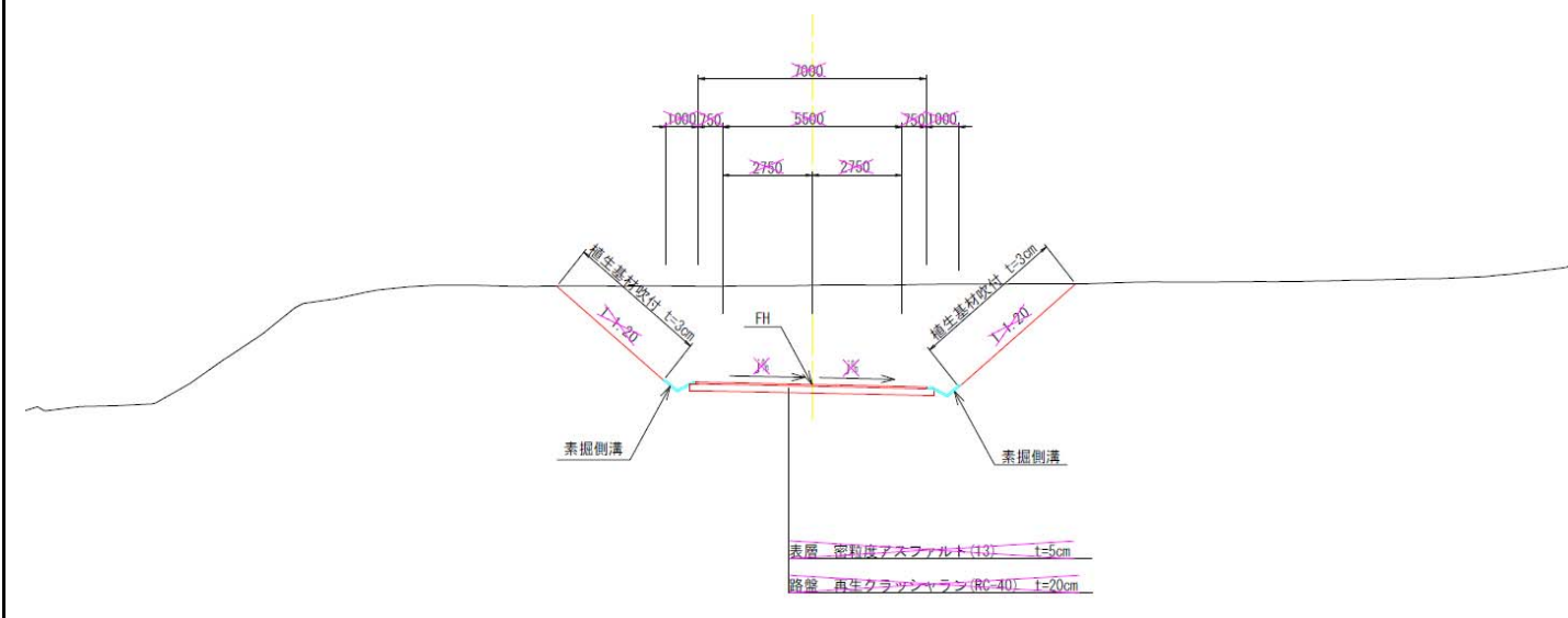
標準断面図(切土部)
