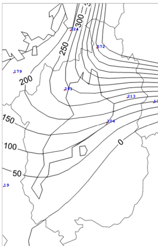
図3 年降雪の深さの合計（平年値：1981～2010年）（単位：cm）
