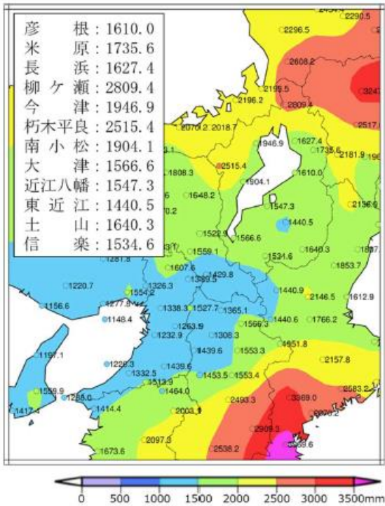
図2 年平均降水量分布図（ 1991～2020 年）（単位：mm）（資料：滋賀県地域防災計画）
