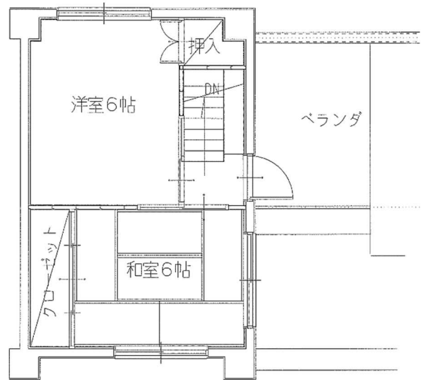
2階建 2階部分
