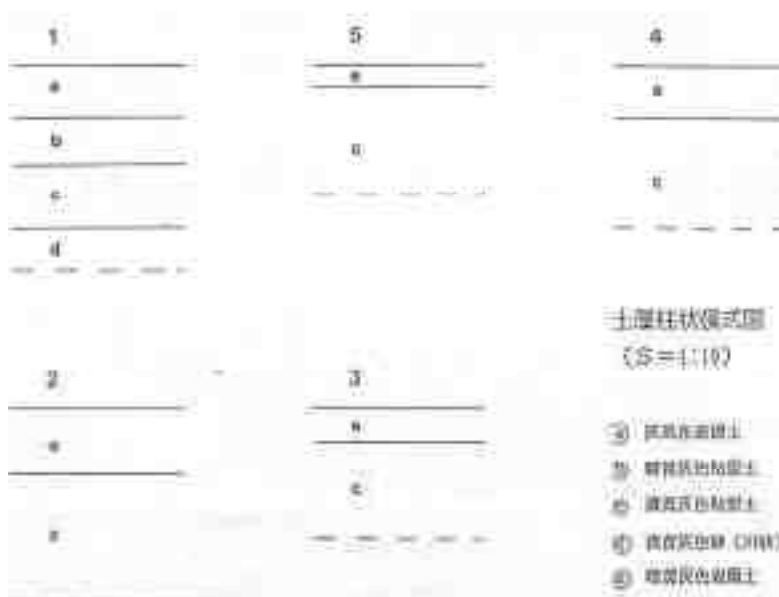
〔図 3-29〕 土層柱状模式図（1：25）
